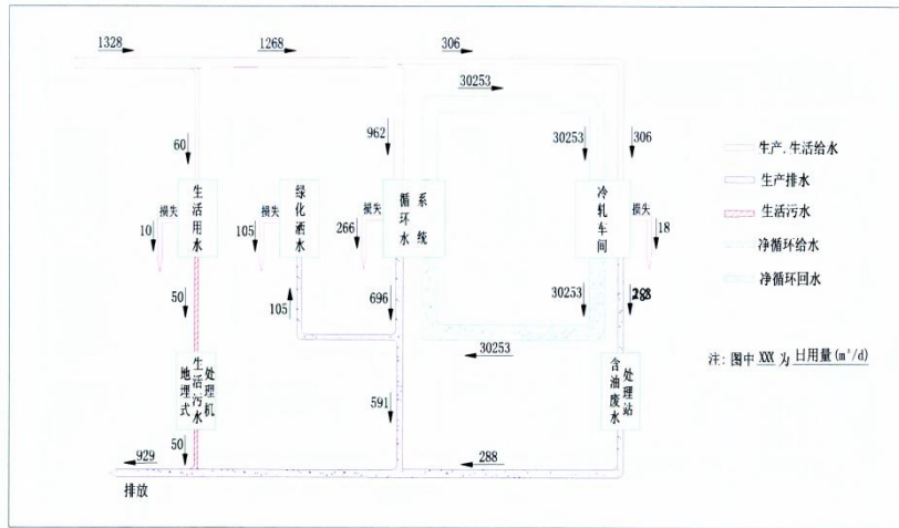
冷轧工程水量平衡图
